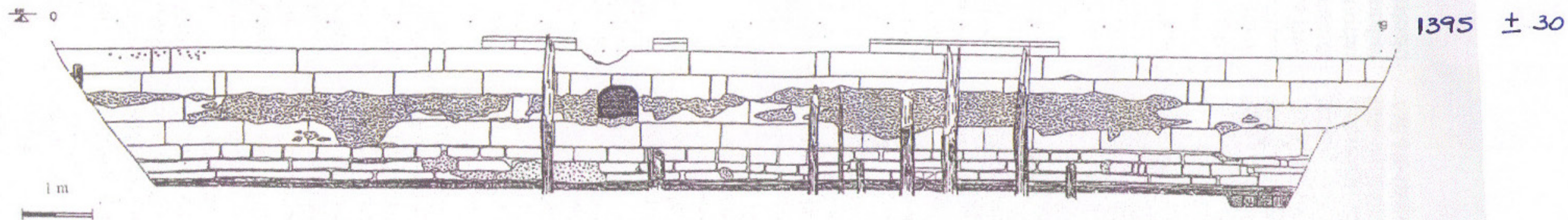
RIALTO (VENEZIA) RIVA SUD COSTRUITA NEL 1398
